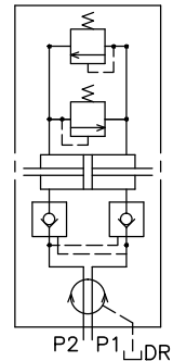
油壓迴路圖
