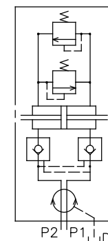
油壓迴路圖
