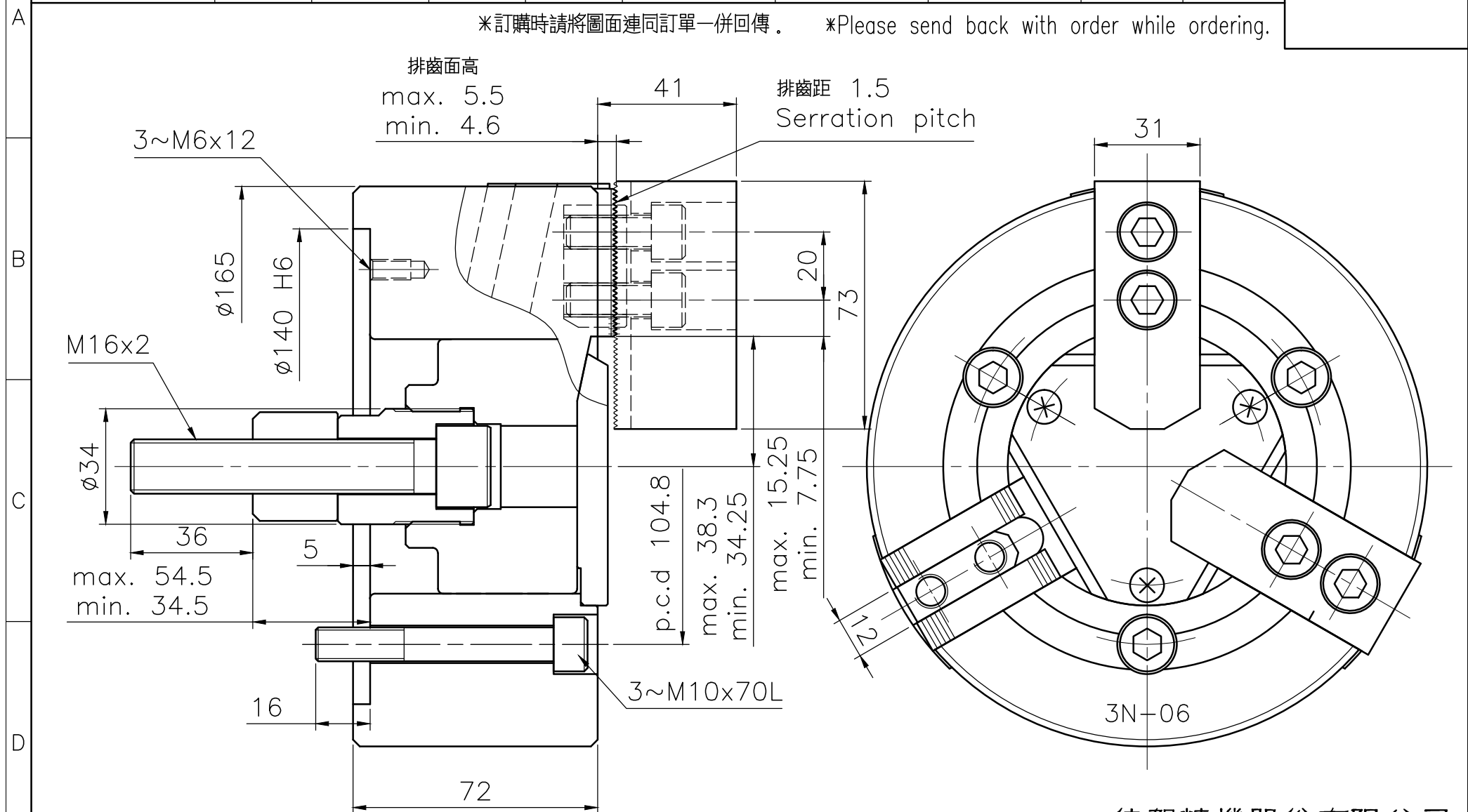
斜爪式中實三爪夾頭
