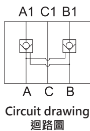
Model:FV-03
