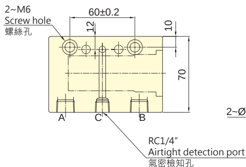
Model:FV-03
