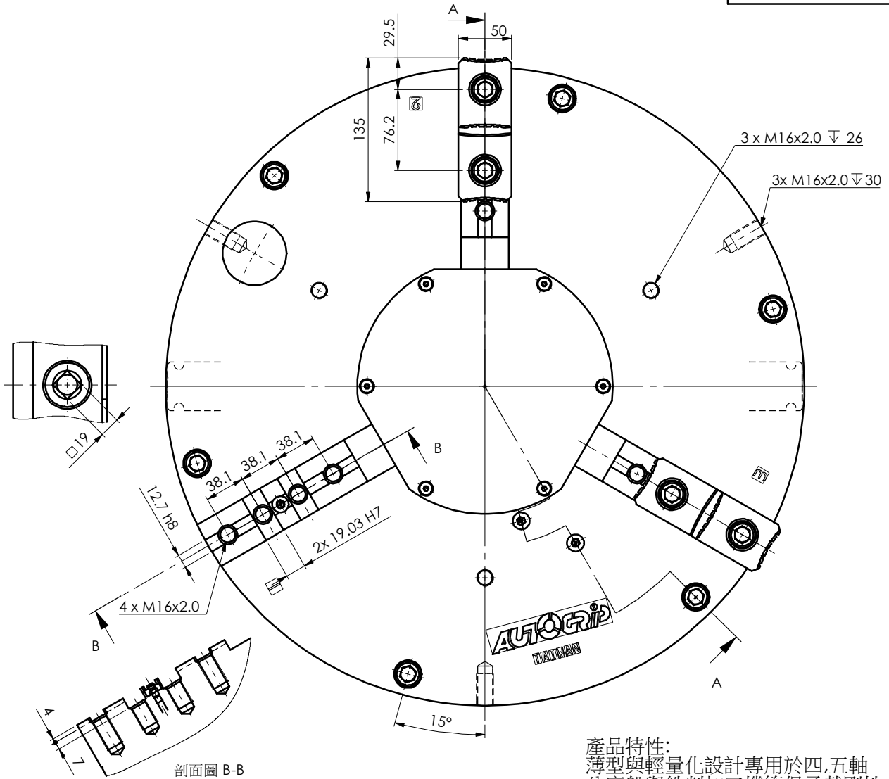
剖面圖 B-B
