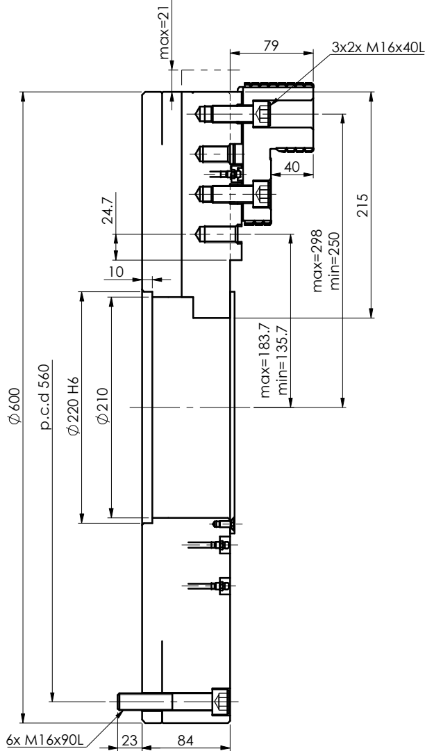
剖面圖 A-A
