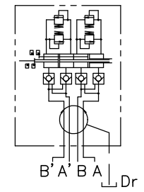
油壓迴路圖
