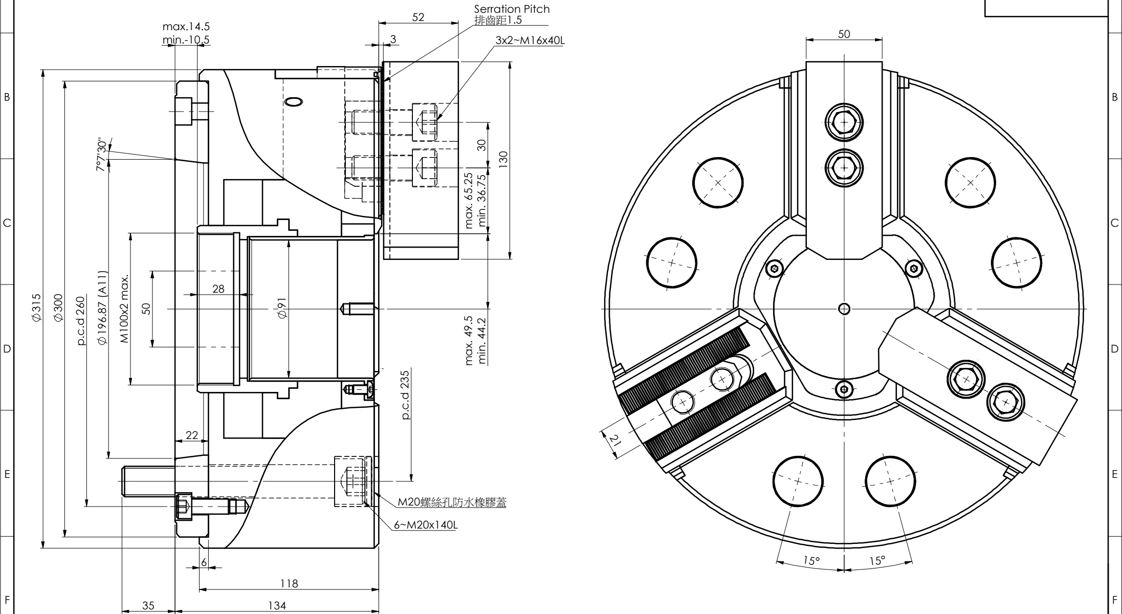
低保養密閉式中空三爪夾頭(A11)
