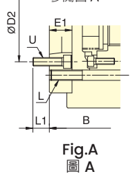
4H-208 A5 4H-210 A6 4H-15 A8 Refer to Fig.A 參閱圖 A
