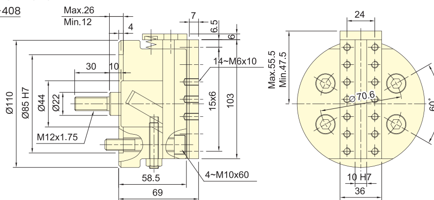
單斜楔式傳動 WEDGE PLUNGER FA-408
