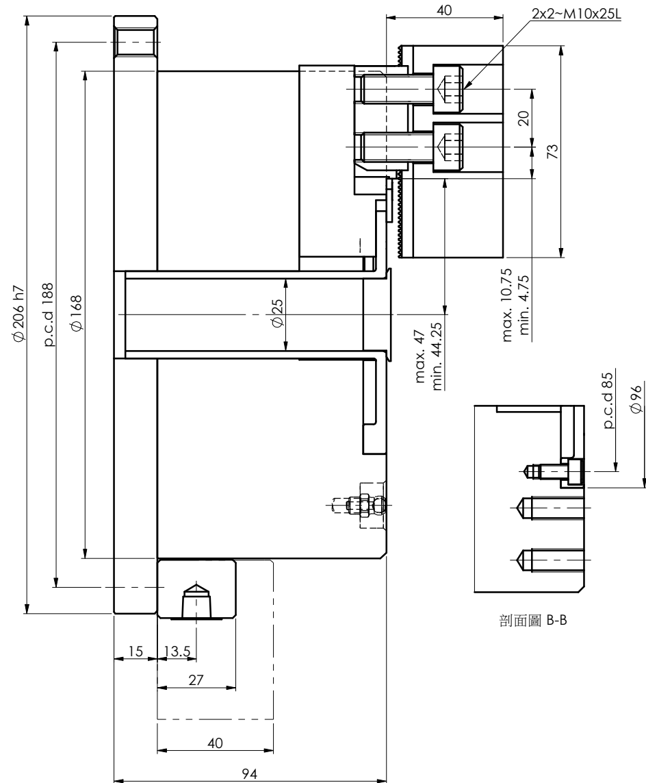
立置式二爪夾頭 剖面圖 A-A
