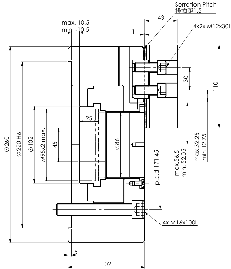
剖面圖 A-A
