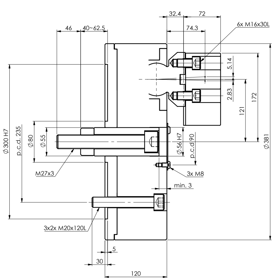
剖面圖 A-A
