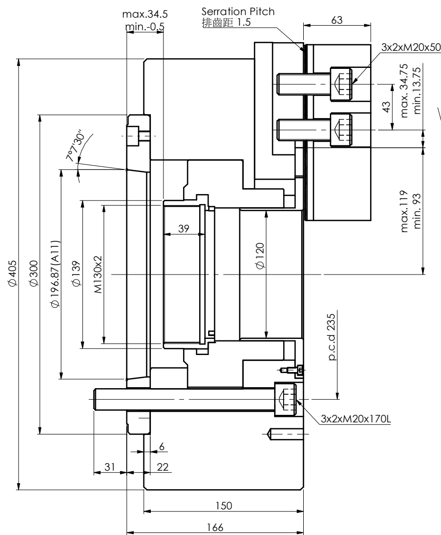
剖面圖 A-A
