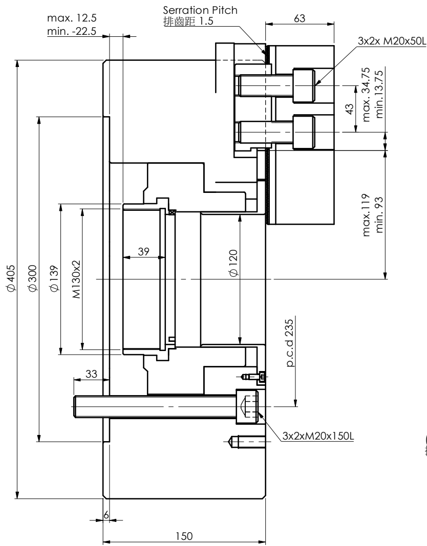
剖面圖 A-A
