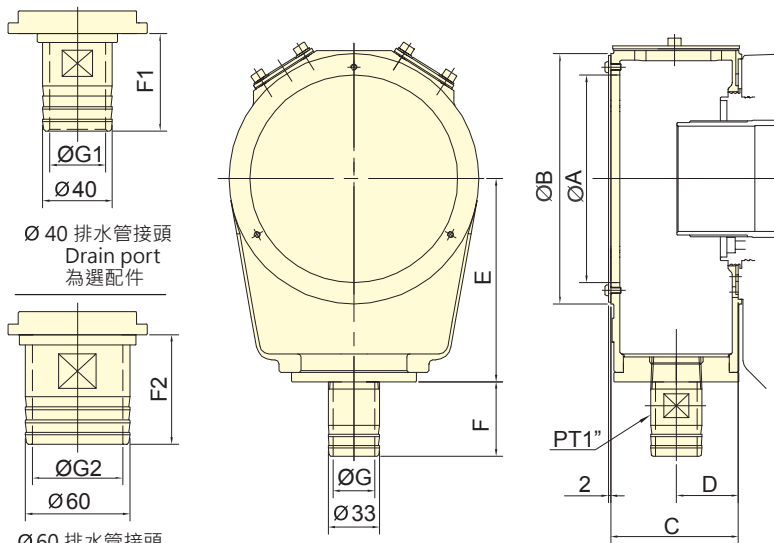
集水盒
